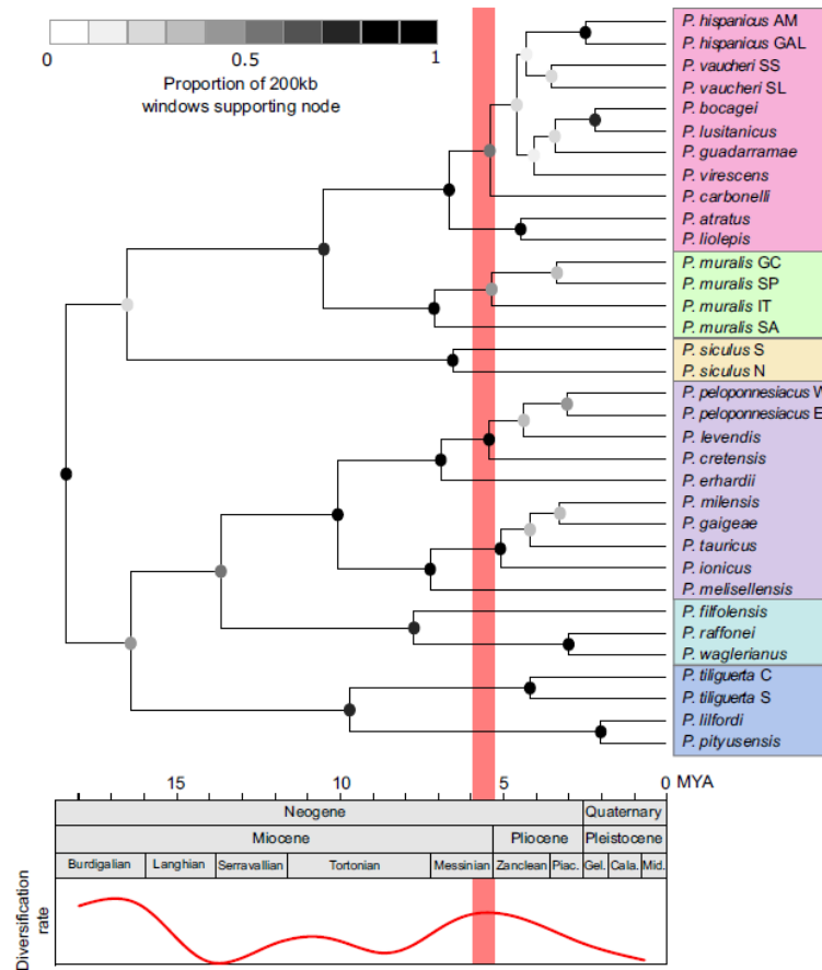
Phylogénie du genre Podarcis à partir de séquences du génome complet (Yang et al. 2021).
