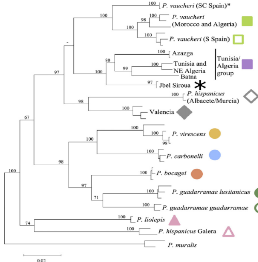
Phylogénie des Podarcis de péninsule Ibérique et d'Afrique du Nord à partir de séquences de l'ADN mitochondrial (Caeiro-Dias 2018, adapté de Kaliontzopoulou et al. 2011).
