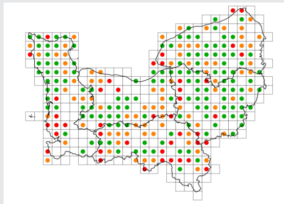
Exemple de la carte de répartition de la Vipère Pélécasse
