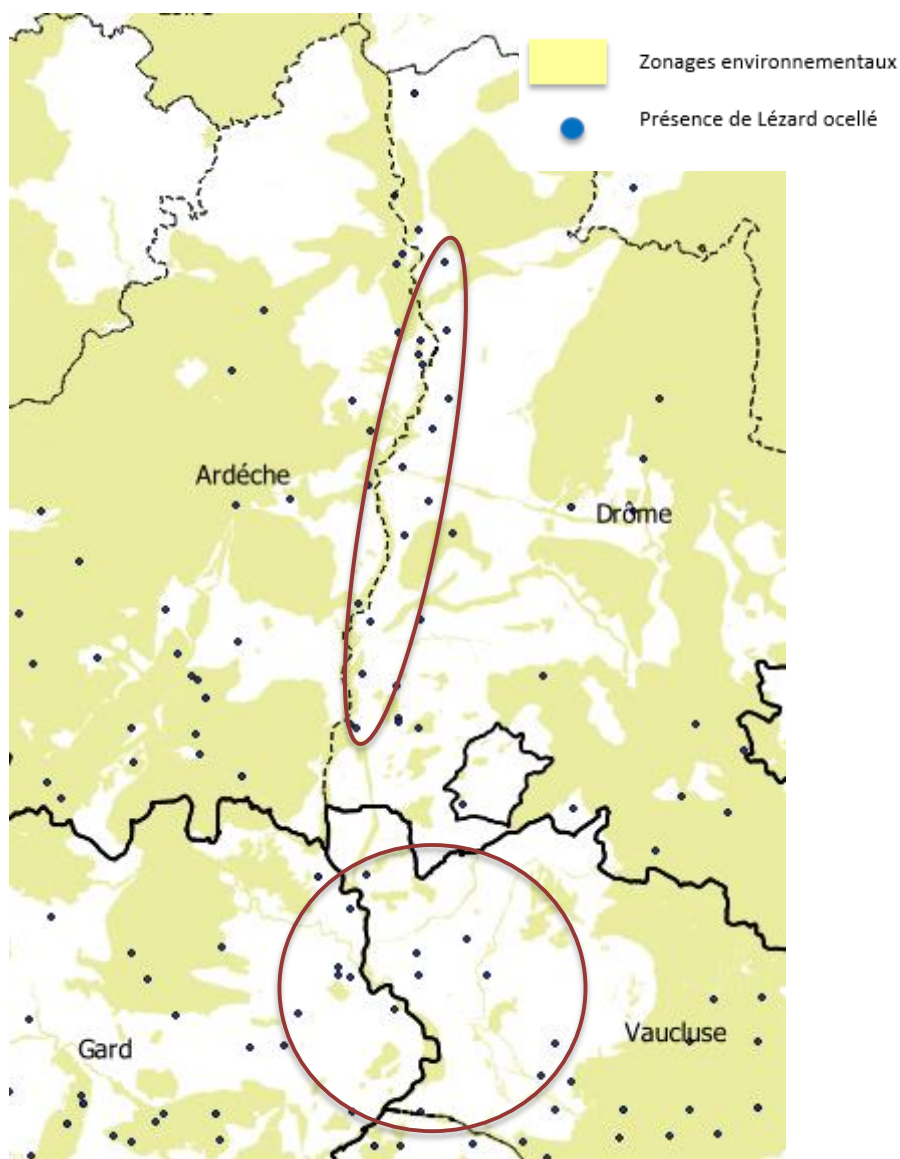
Figure 29. Zoom sur le prise en compte du Lézard ocellé dans les zonages environnementaux dans les départements du Gard, de l'Hérault et de la Drôme
