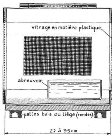
COUPE TRANSVERS.
